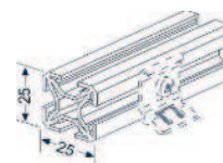
Монтажный профиль
