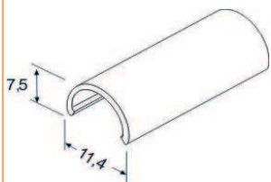
Декоративный алюминиевый профиль белый, темно-коричневый, латунь, металлик
