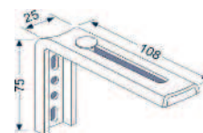
Выносной кронштейн 100-150мм для F4, FE
