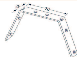
Соединительный кронштейн белый, серый, черный
