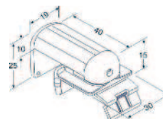
Кронштейн «без сверления» для F4, FE белый, черный, серый
