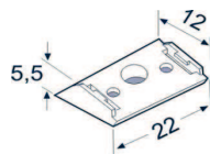
Клинышек 15° белый, черный
